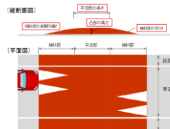
ハンプの構造
