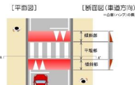
スムーズ横断歩道の構造
